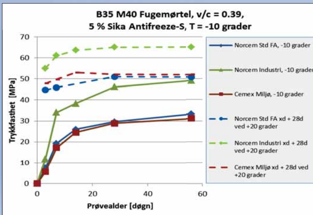
Figur 6: Fasthetsutvikling ved -10 grader for B35 M40 fugebetong med de mest aktuelle norske sementene. Alle fugebetongene er tilsatt 5 % Sika Antifreeze-S (Natriumnitrat, pulver). «Heltrukne» kurver viser fasthet for prøver lagret x døgn ved -10 grader. «Stiplede» kurver viser fasthet for prøver lagret x døgn ved -10 grader og deretter vannlagret ved +20 grader i 28 døgn før trykking.
